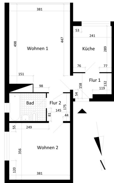
Grundriss
