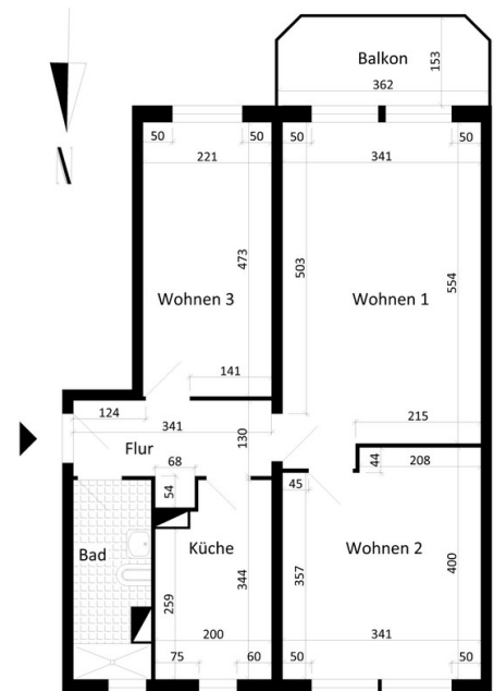
Grundriss
