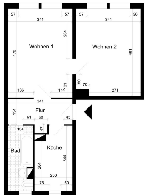
Grundriss
