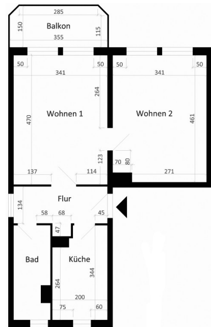
Grundriss mit Balkon
