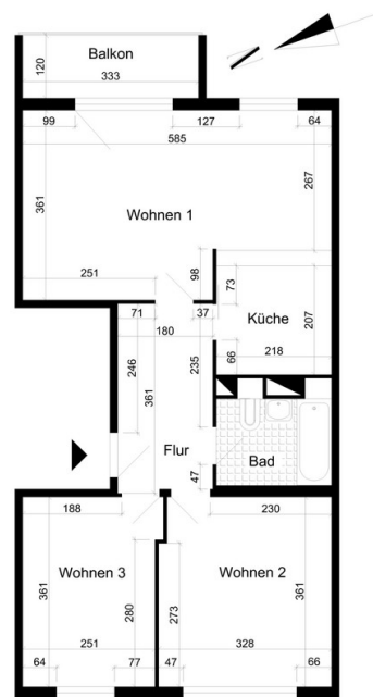
Grundriss
