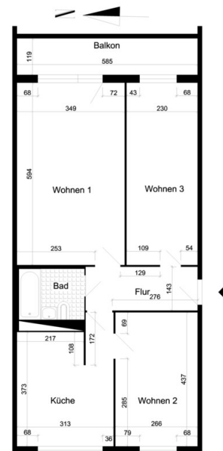
Grundriss
