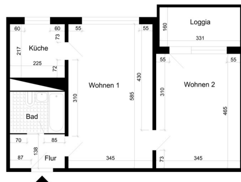
Grundriss
