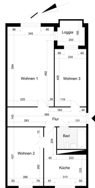
Grundriss
