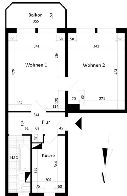
Grundriss
